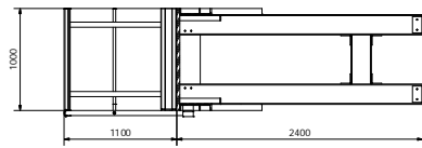
D-D (1 : 20)
