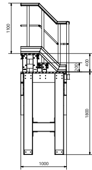
B-B (1 : 20)
