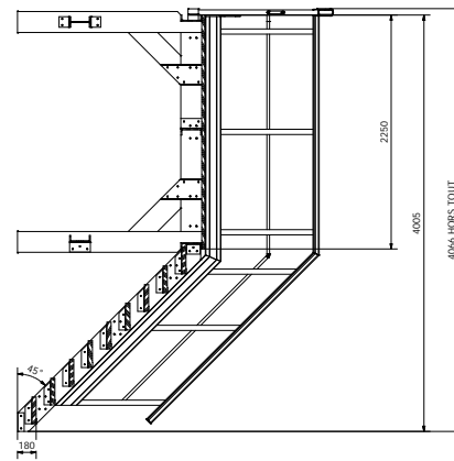
C-C (1 : 20)
